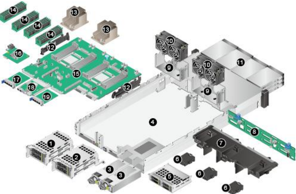
图 4-20 部件
