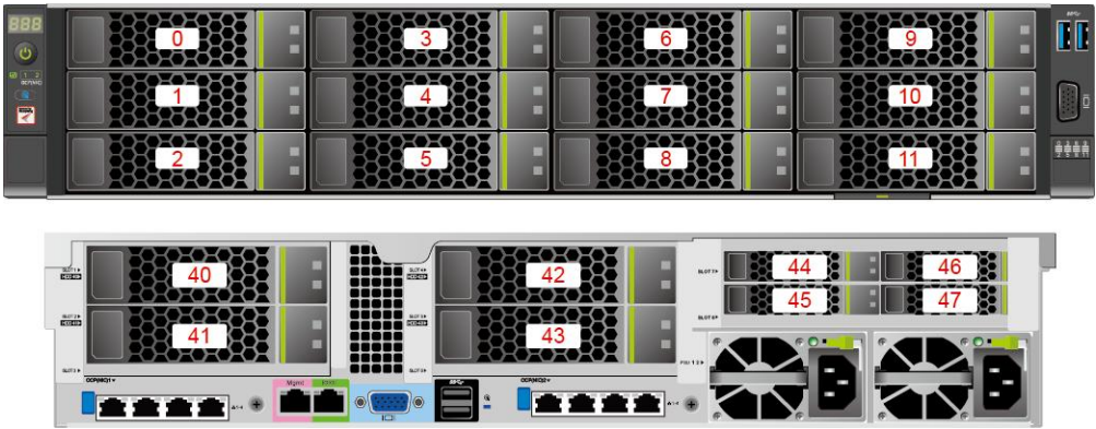
图 6-3 12x3.5 英寸 EXP 硬盘配置
